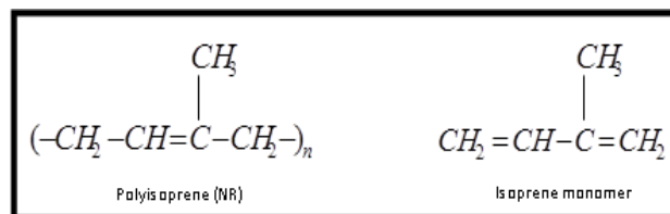
Fig .1 : Isoprene units
